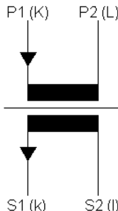
Schaltbild / connection diagram:
