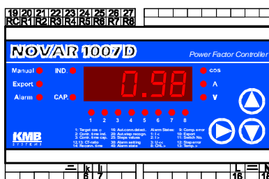
Рис. 2.5 : Регулятор Novar-1007D
